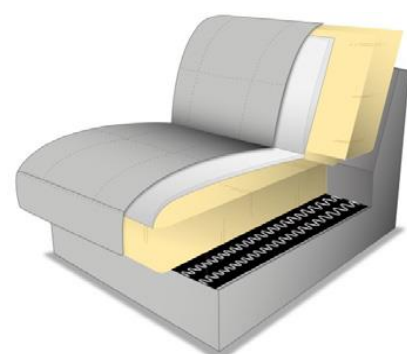
PUR - pěna na vlnovcových pružinách (STANDARD)
