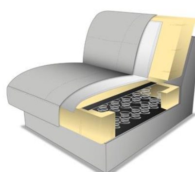
Pružinový sedák (za příplatek)
